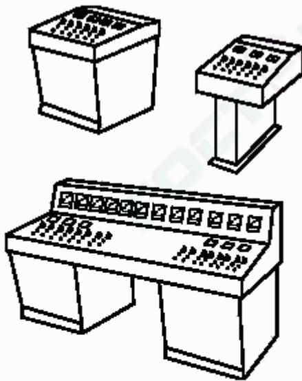
Рисунок С.5 — НКУ заводского изготовления пультового типа
