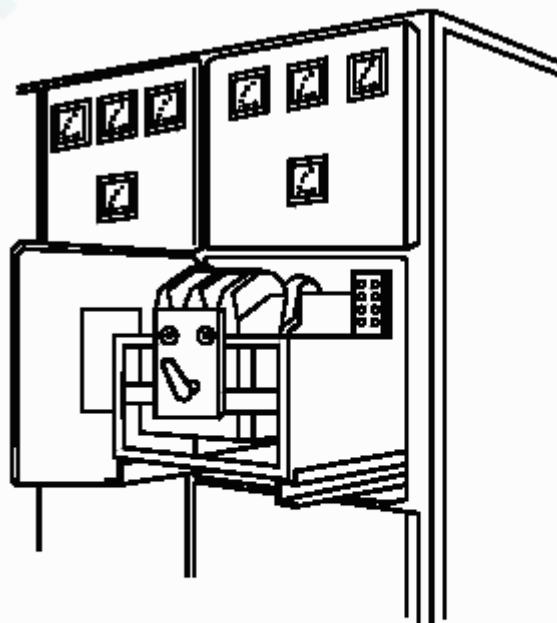
Рисунок С.10 — Выдвижная часть
