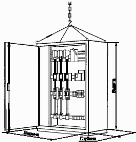
Рисунок С.3 — НКУ заводского изготовления шкафного типа
