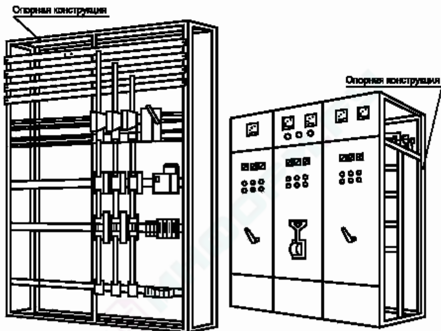
Рисунок С.1 — НКУ заводского изготовления открытого типа
