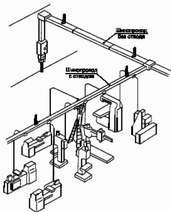
Рисунок С.7 — Система сборных шин (шинопровод)
